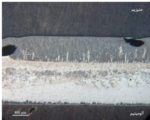
شکل ۶- تصویر میکروسکوپی نوری از نمونه ریخته‌گری شده در سرعت دوران ۱۶۰۰ دور بر دقیقه
