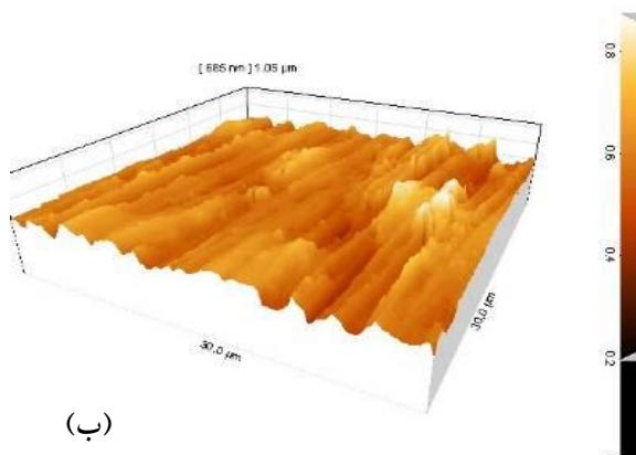
شکل ۸- تصویر میکروسکوپی نیروی اتمی از سطح آلومینیم: (الف) تصویر دو بعدی سطح و (ب) تصویر سه بعدی سطح
