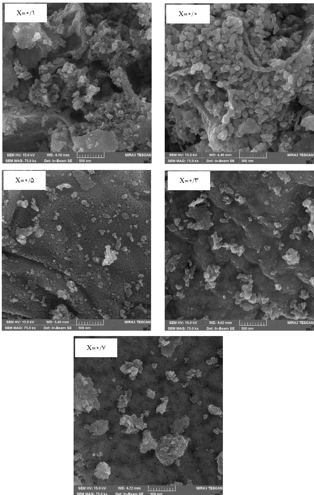
شکل ۳- تصاویر میکروسکوپی الکترونی روبشی نمونه‌های فریت کبات آرایش یافته با کروم به‌ازای درصدهای مختلف آرایش
