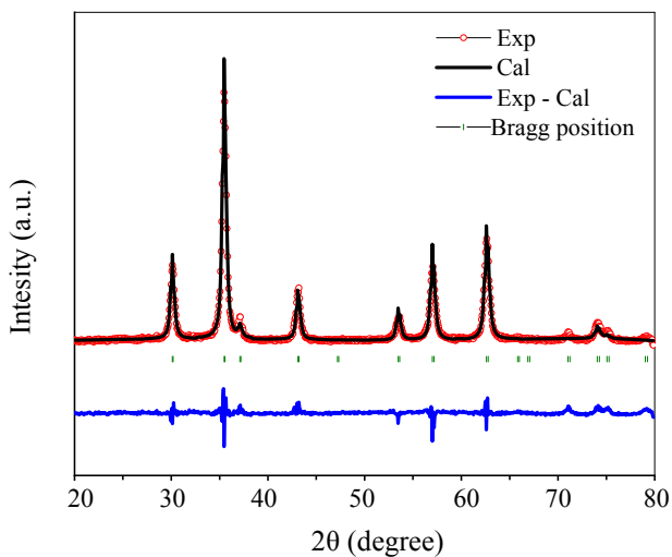
شکل ۲- تحلیل ریتولد نمونه Co_{0.5}Zn_{0.5}Fe_{1.5}Cr_{0.5}O_4
