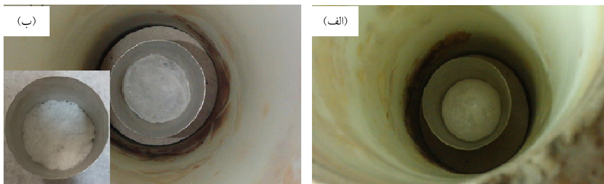
شکل ۲- تصاویر نمونه \text{CaB}_4\text{O}_7 تحت فرایند حرارتی: الف) شروع خروج گازها از نمونه در دمای ۲۲۴ درجه سانتی‌گراد و ب) بازگشت حباب به محتویات داخل بوتله در دمای ۲۸۰ درجه سانتی‌گراد (تصویر موجود در ضمیمه، نمونه را پس از اتمام فرایند حرارتی نشان می‌دهد)
