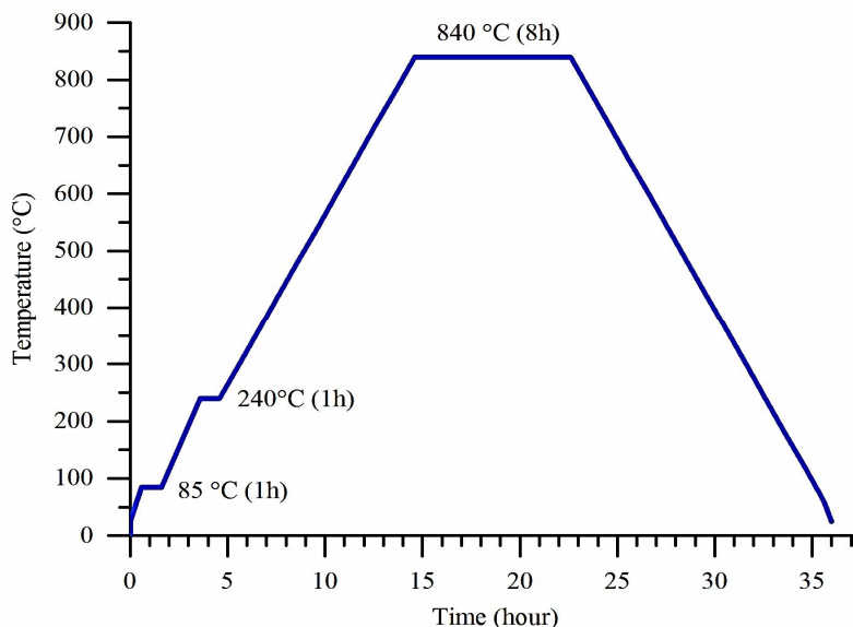
شکل ۱- نمودار دما - زمان فرایند سنتز نمونه‌های \text{CaB}_4\text{O}_7
