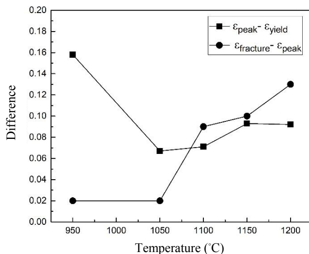
شکل ۸- بررسی اختلاف بین کرنش نقطه حداکثر و تسلیم ( \epsilon_{\text{yield}} - \epsilon_{\text{peak}} ) و نقطه شکست و حداکثر ( \epsilon_{\text{fracture}} - \epsilon_{\text{peak}} ) برای آلیاژ 25 Haynes در دماهای مختلف آزمایش
