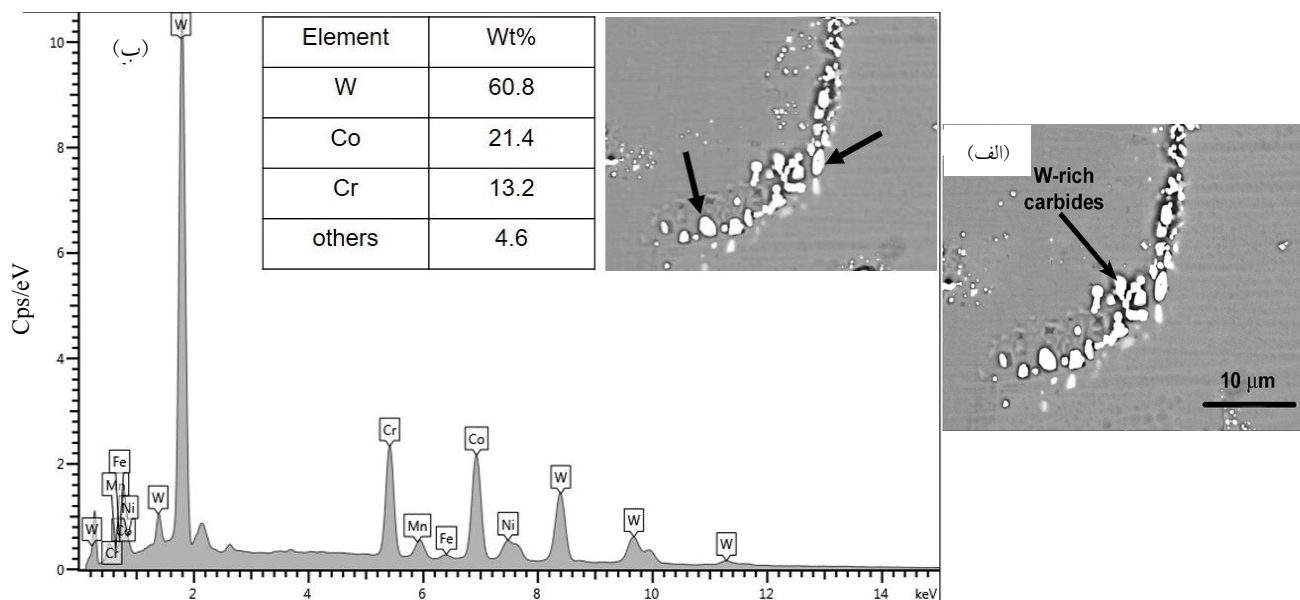
شکل ۵- (الف) ریزساختار میکروسکوپی الکترونی روبشی از آلیاژ Haynes 25 در حالت ریختگی و همگن شده و (ب) آنالیز طیف پراش انرژی از ذره نشان داده شده
