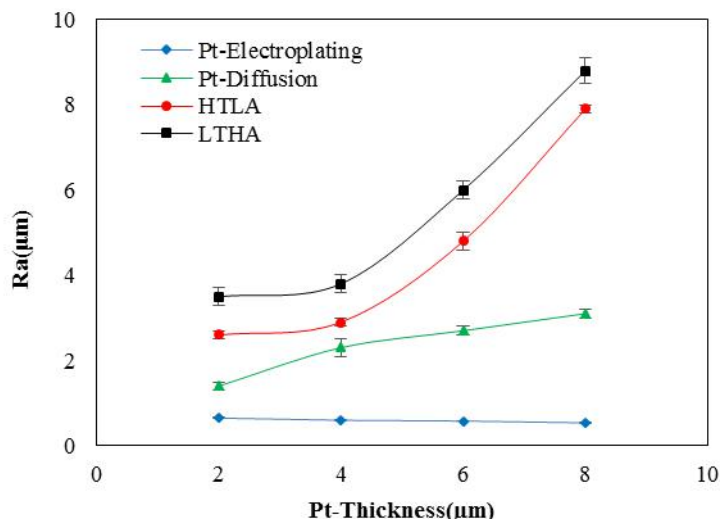
شکل ۱۳- تغییرات زبری سطح در مراحل مختلف پوشش دهی و در ضخامت های مختلف از پلاتین اولیه
