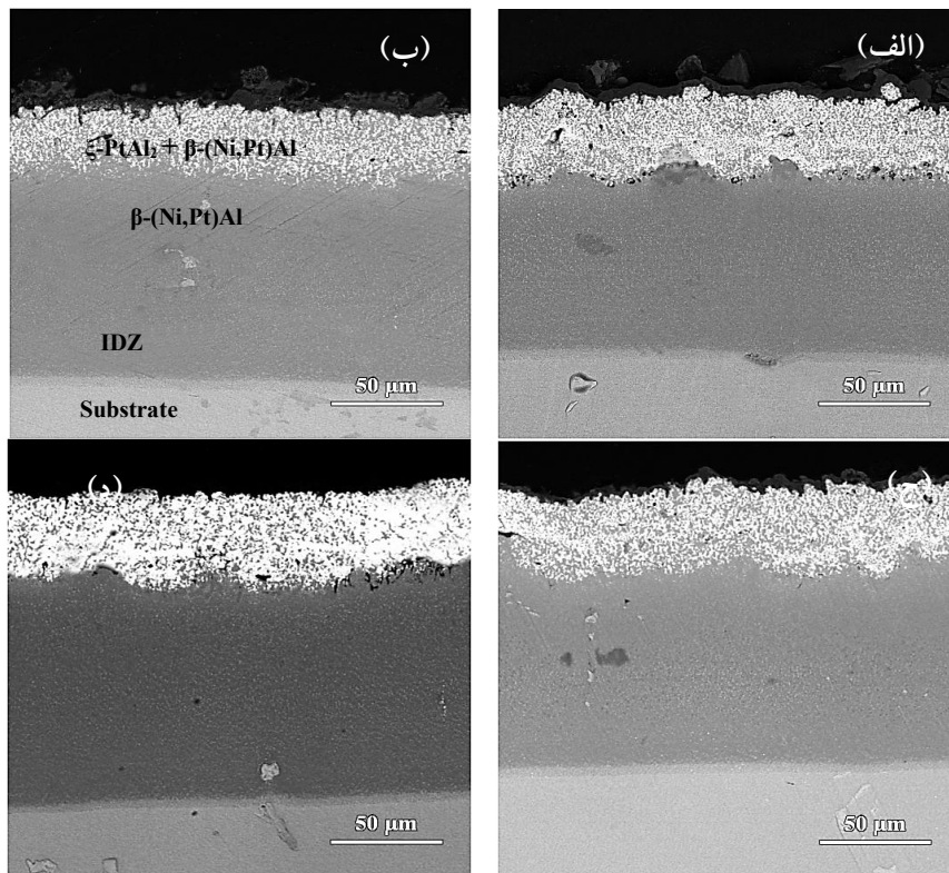
شکل ۵- تصاویر میکروسکوپی الکترونی روبشی (الکترون برگشتی) از پوشش پلاتین-آلومیناید در شرایط LTHA برای ضخامت‌های: الف) ۲، ب) ۴، ج) ۶ و د) ۸ میکرومتر از پلاتین
