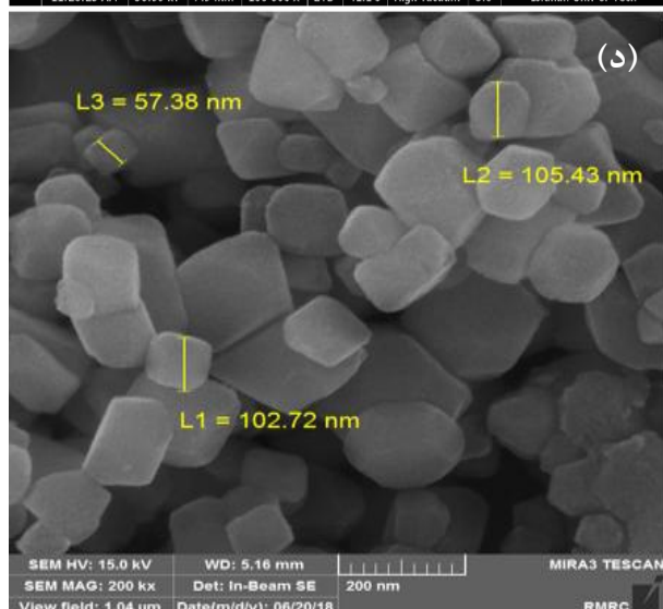
شکل ۴- تصاویر میکروسکوپی الکترونی روبشی گسیل میدانی لیتیم فلورید سنتز شده در دمای: الف و ب) ۳۰۰ و ج و د) ۴۰۰ درجه سانتی‌گراد
