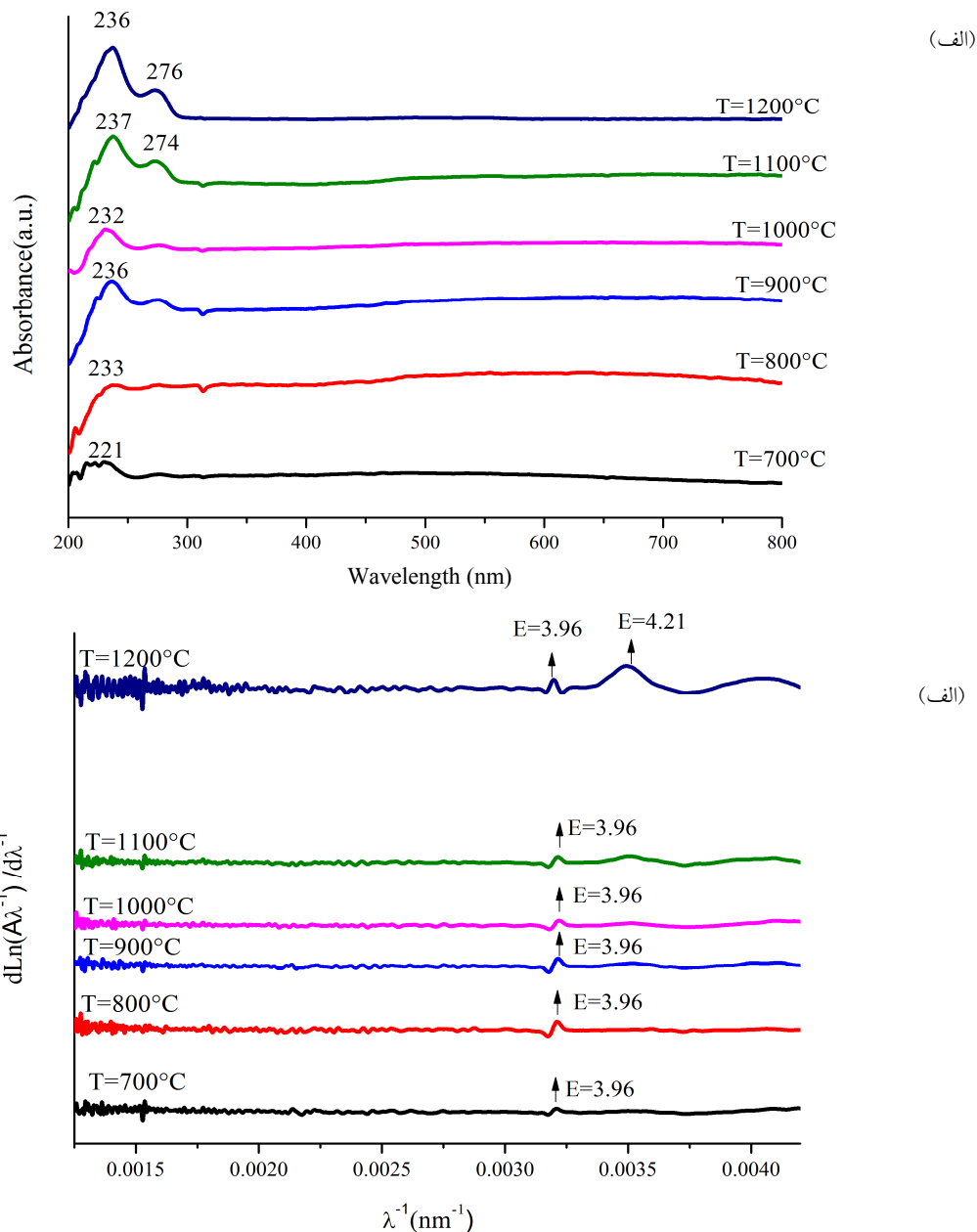
شکل ۶- الف) منحنی‌های جذب بر حسب طول موج و ب) نمودار dLn(A\lambda^{-1})/d\lambda^{-1} بر حسب \lambda^{-1} برای نانوساختارهای SrCo_2Fe_{16}O_{27} با دماهای مختلف
