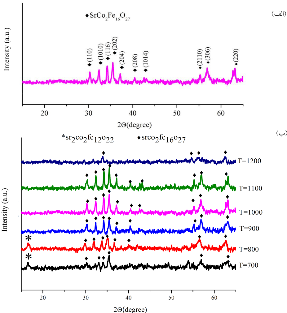
شکل ۲- الف) الگوی پراش پرتو ایکس نانو ساختار SrCo_2Fe_{16}O_{27} در دمای ۱۰۰۰ درجه سانتی گراد و ب) الگوی پراش پرتو ایکس نانو ساختار SrCo_2Fe_{16}O_{27} در دماهای مختلف
