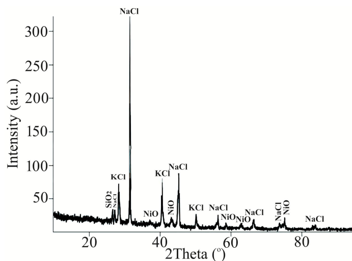
شکل ۷- الگوی پراش پرتو ایکس از سطح نمونه پس از آزمون خوردگی فرسایشی دامبالا در شرایط R3
