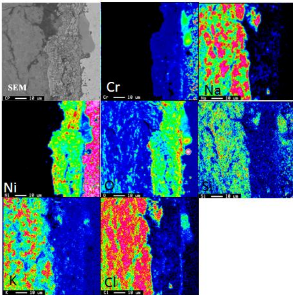
شکل ۶- نقشه توزیع عناصر آلیاژی (EDS mapping) نمونه پس از آزمون خوردگی فرسایشی دامبالا در شرایط R3
