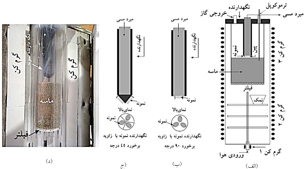
شکل ۱- طرح‌واره: الف) دست‌چاه آزمون خوردگی فرسایشی دما بالا، ب) نگهدارنده نمونه با زاویه برخورد عمودی، ج) نگهدارنده نمونه با زاویه برخورد ۴۵ درجه و د) تصویر محفظه واکنش نمونه
