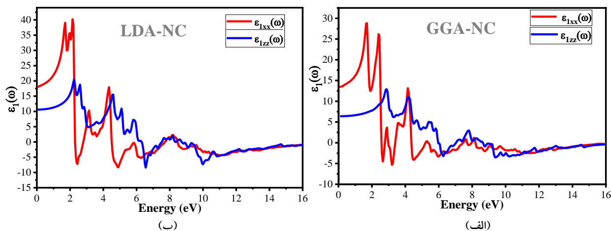
شکل ۲- تغییرات سهم حقیقی تابع دی‌الکتریک نسبت به انرژی فوتون‌های فرودی در راستای x و z در تقریب‌های الف) GGA-NC و ب) LDA-NC (رنگی در نسخه الکترونیکی)
