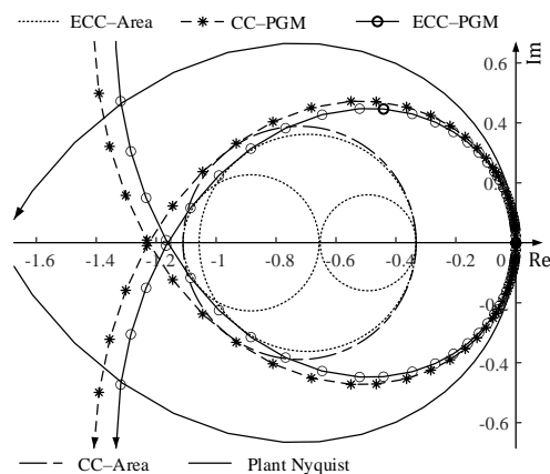
شکل ۱۴. حد بهره سیستم حلقه بسته (\Sigma_3, l_{\psi_3}(0.9, 3)) با معیار CC و ECC.
