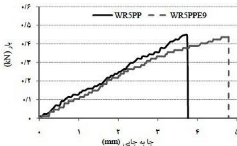
شکل ۳. رفتار بار- جابه‌جایی مواد مرکب آرد چوب- پلی پروپیلن پنج‌بار بازیافتی
