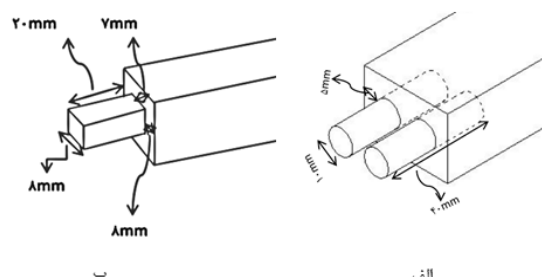
شکل ۲. ابعاد و طرح اتصالات: الف- پین چوبی، ب- ابعاد زبانه
