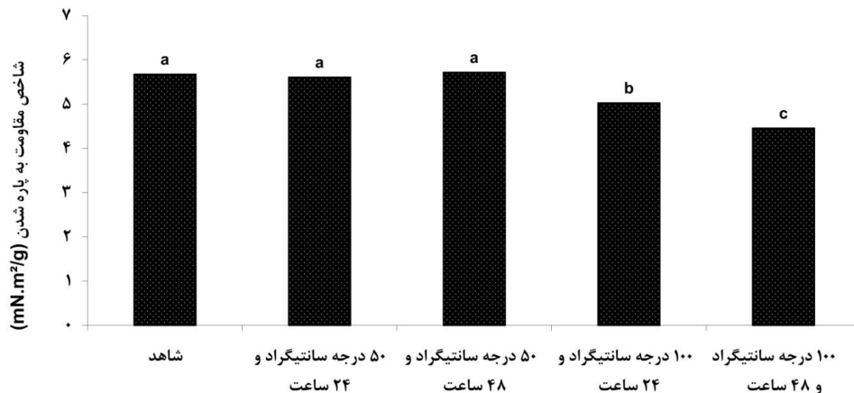
شکل ۴. تأثیر کهنگی تسریع شده حرارتی بر شاخص مقاومت به پاره شدن
