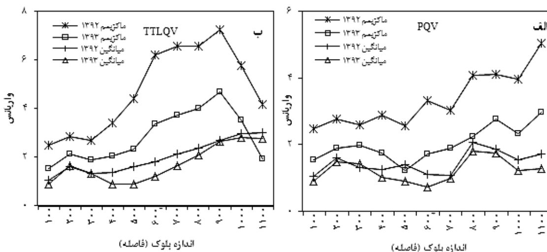
شکل ۲. نتایج تجزیه و تحلیل داده‌ها برای تشخیص الگوی پراکنش خشکیدگی تاج در درختان بلندمازوی آلوده به بیماری پوسیدگی زغالی: (الف) PQV تجزیه و تحلیل میانگین و ماکزیمم داده‌ها در دو سال؛ (ب) TILQV تجزیه و تحلیل میانگین و ماکزیمم داده‌ها در دو سال.
