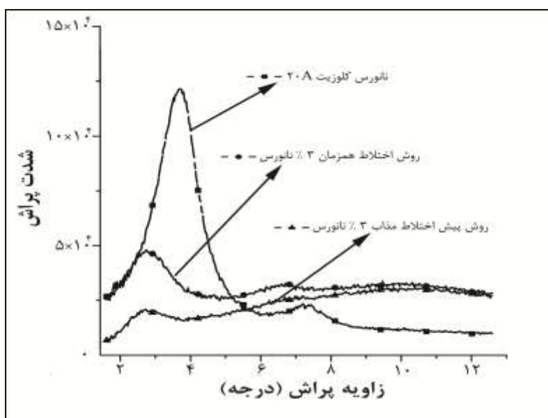
شکل ۱. الگوی پراش اشعه ایکس نانورس خالص و چندسازه‌های چوب پلاستیک ساخته‌شده به روش اختلاط همزمان و پیش‌اختلاط
