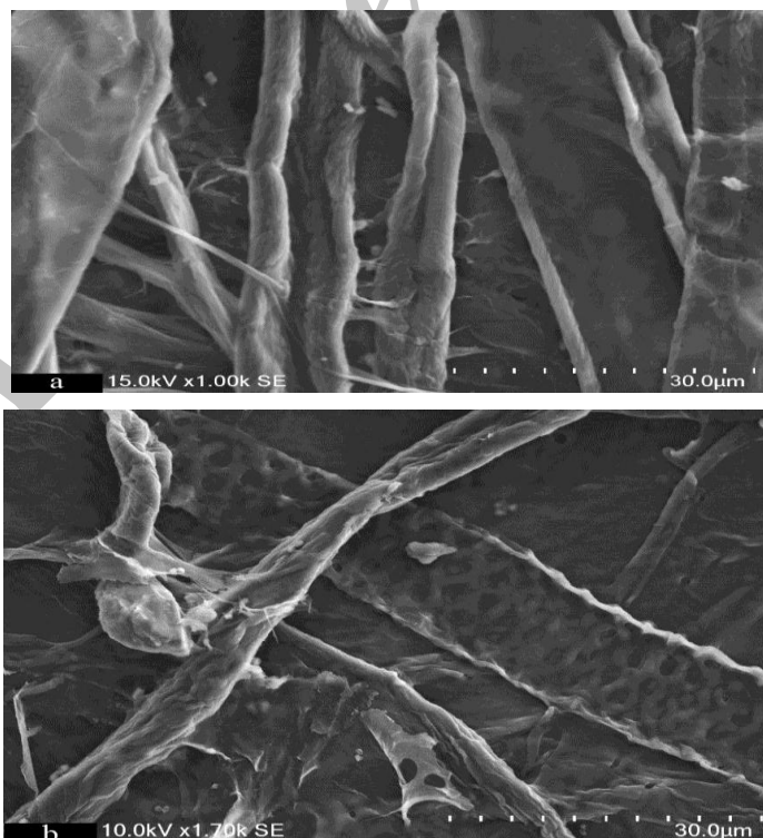
شکل ۲. تصاویر میکروسکوپ الکترونی روبشی نمونه کاغذ باگاس و نانوالیاف سلولزی کاتیونی (a) و کاغذ باگاس و نانوالیاف سلولزی - نشاسته کاتیونی (b) با بزرگنمایی ۱۸۰۰ برابر
