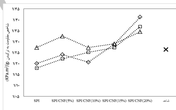
شکل ۱. شاخص مقاومت به ترکیدن کاغذهای پوشش‌داده شده با درصد‌های مختلف نانوالیاف سلولزی و ایزوله پروتئین سویا (SPI/CNF) در وزن‌های پوشش ۵ ( \diamond ), ۱۰ ( \square ) و ۱۵ ( \triangle ) g/m^2
