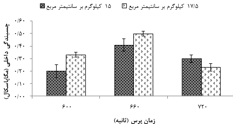
شکل ۱. اثر متقابل زمان و فشار پرس بر چسبندگی داخلی تخته‌های ساخته‌شده با آرد ذرت / آرد کنجاله سویا
