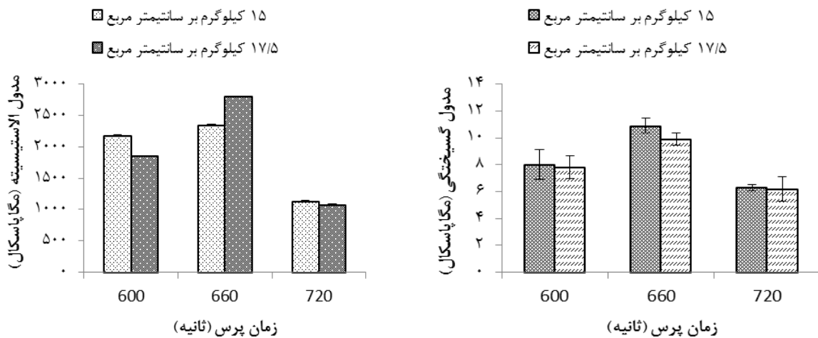
شکل ۲. اثر متقابل زمان و فشار پرس بر ویژگی‌های خمشی تخته‌های ساخته‌شده با آرد ذرت / آرد کنجاله سویا
