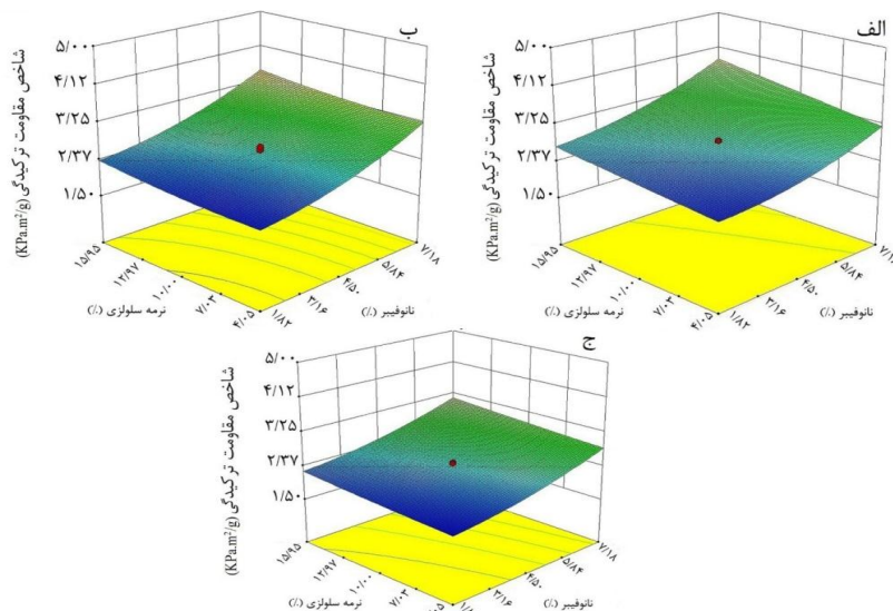
شکل ۲. اثر کاربرد نانوفیبر و نرمه‌های کاغذسازی به همراه سه نوع ماده کاتیونی (الف: نشاسته کاتیونی، ب: PAC و ج: CPAM) بر شاخص مقاومت ترکیبی کاغذ حاصل از الیاف بازیافتی
