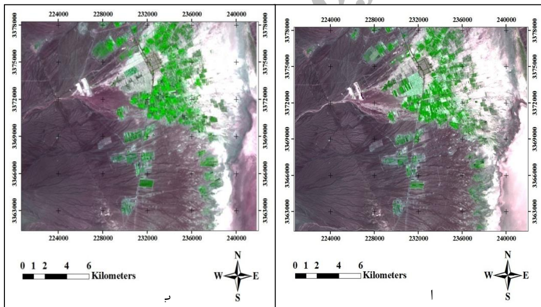
شکل ۵. محدوده مورد مطالعه در ترکیب باندهای ۱، ۲، ۳، و ۱ تصویر ASTER: الف) سال ۲۰۰۳؛ ب) سال ۲۰۱۰
