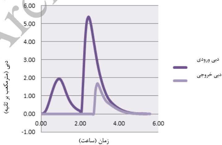
شکل ۷. مقایسه هیدروگراف ورودی و خروجی سازه ۷
