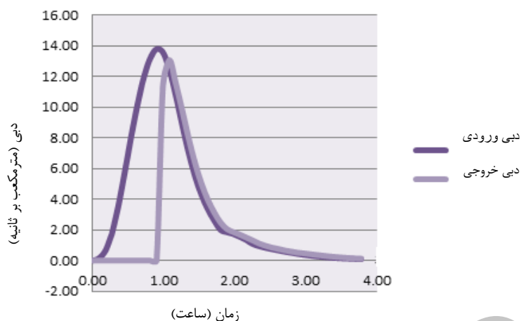
شکل ۷. مقایسه هیدروگراف ورودی و خروجی سازه ۷
