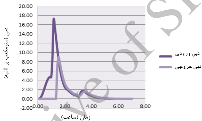
شکل ۹. مقایسه هیدروگراف ورودی و خروجی سازه ۹
