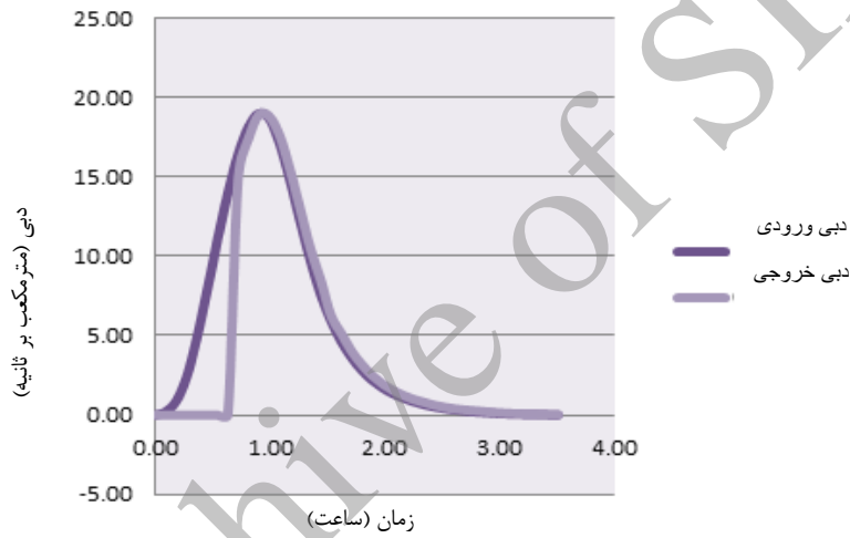
شکل ۴. مقایسه هیدروگراف ورودی و خروجی سازه ۲
