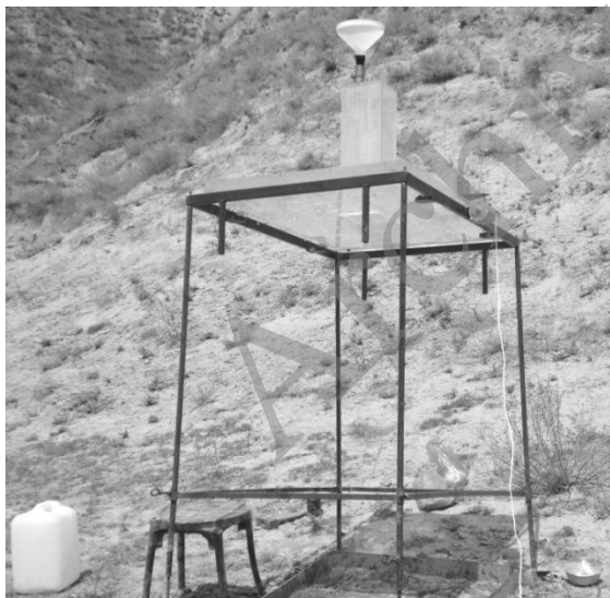
شکل ۲. دستگاه شبیه‌ساز باران مورد استفاده در این پژوهش
