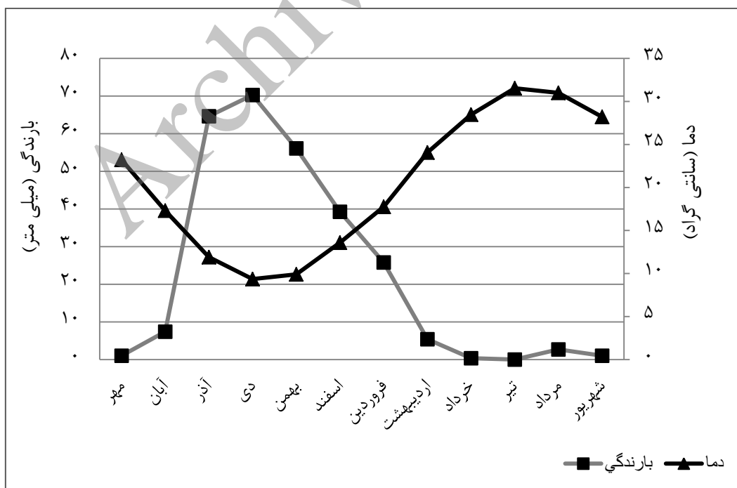
شکل ۶. نمودار آمبروترمیک ایستگاه هواشناسی جهرم (۱۳۵۹ - ۱۳۹۲)
