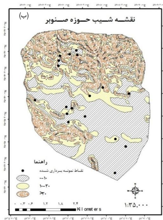
شکل ۲. نقشه واحدهای زمین‌شناسی (الف) و شیب (ب) و نقاط نمونه‌برداری شده حوزه صنوبر
