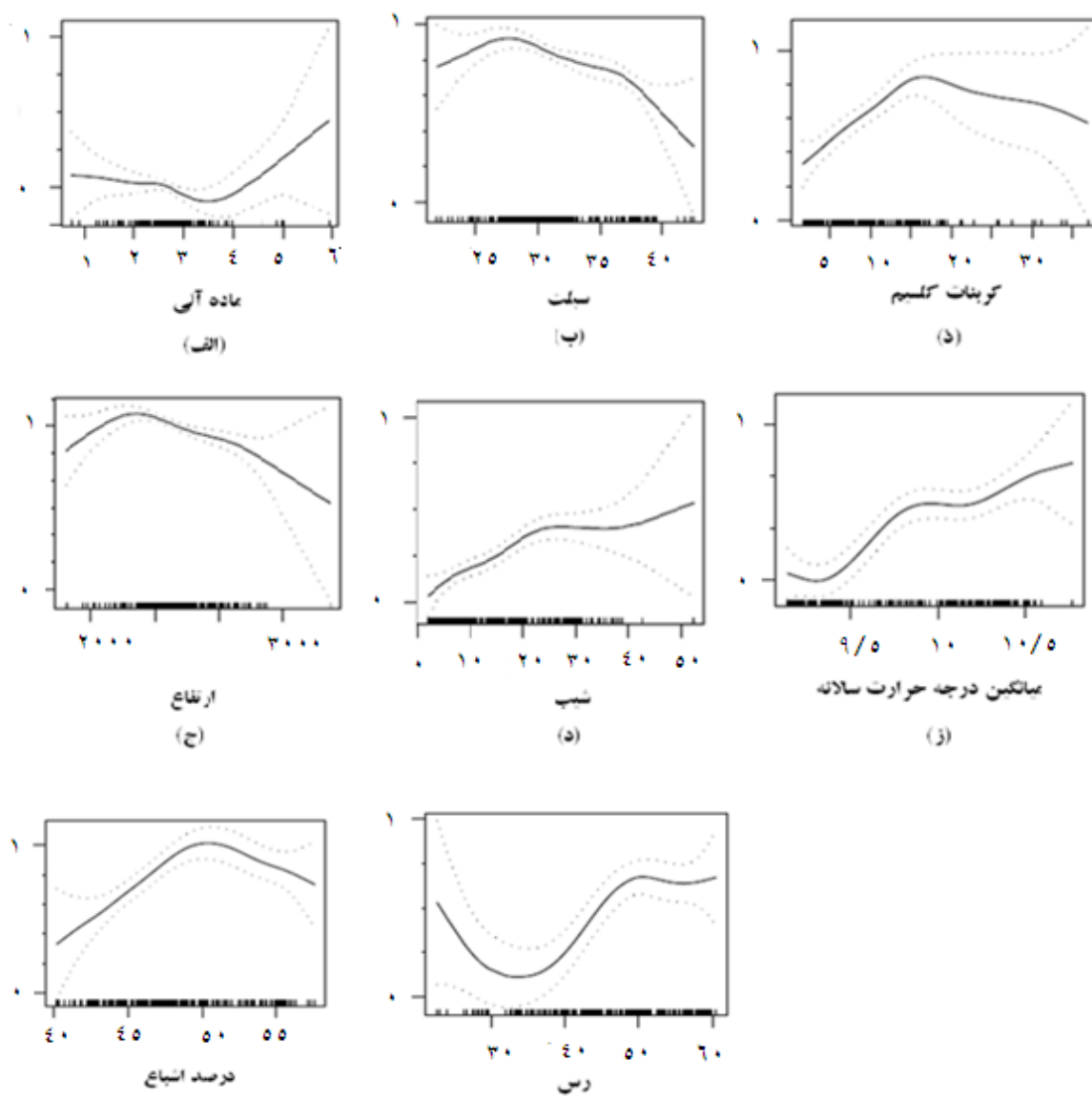
شکل ۵- منحنی عکس‌العمل متغیرهای محیطی (اقلیمی، خاک و فیزیوگرافی) در منطقه مورد مطالعه می‌باشد. خط پر رنگ نشان‌دهنده احتمال رخداد گونه نسبت به متغیر محیطی و خطوط خط چین نشان‌دهنده فاصله اطمینان ۹۵ درصد می‌باشد. متغیر دما بر حسب درجه سانتیگراد، ارتفاع از سطح دریا بر حسب متر و سایر متغیرها بر حسب درصد ارایه شده است.
