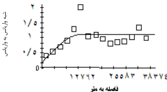
شکل ۲- مدل واریوگرام تولیدشده درصد رس
