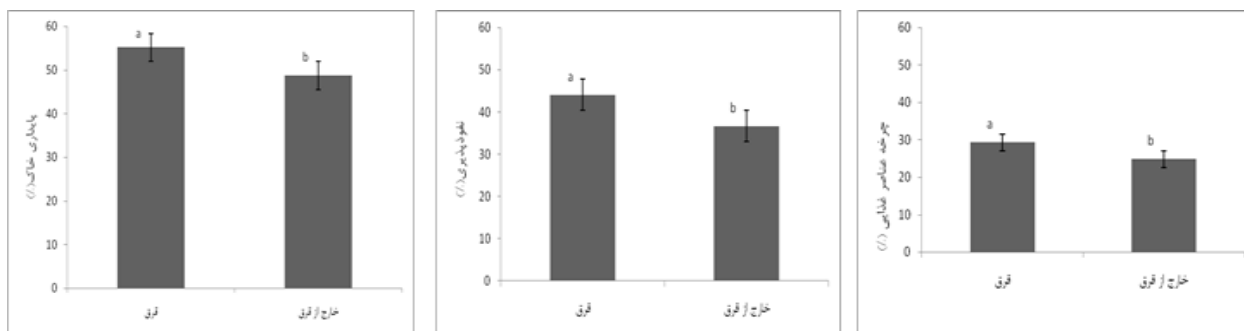
شکل ۱. مقایسه ویژگی‌های عملکردی شاخص‌های سطح خاک در دو منطقه قرق و خارج قرق مراتع دونا
