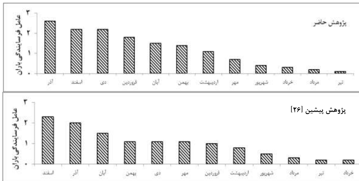
شکل ۲. اولویت‌بندی ماه‌های مختلف از نظر خطر عامل فرساینده‌گی باران (تن متر سانتی متر بر هکتار ساعت) در کشور طی پژوهش حاضر (بالا) و پیشین [۲۶] (پایین).
