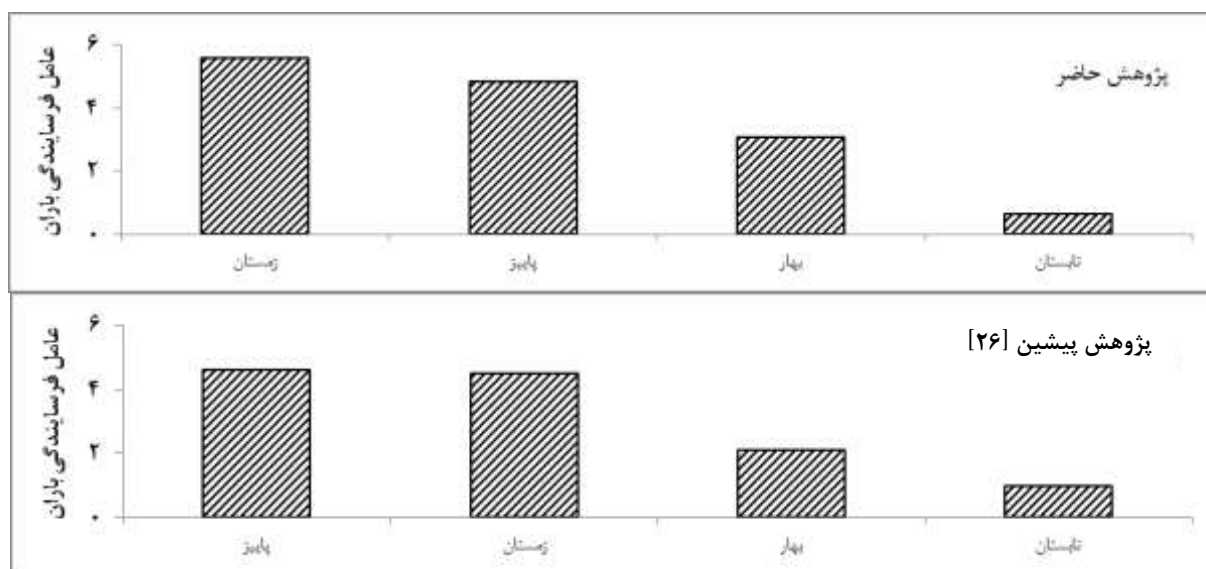
شکل ۳. اولویت‌بندی فصل‌های مختلف از نظر خطر عامل فرساینده‌گی باران (تن‌متر سانتی‌متر بر هکتار ساعت) در کشور طی پژوهش حاضر (بالا) و پیشین [۲۶] (پایین).
