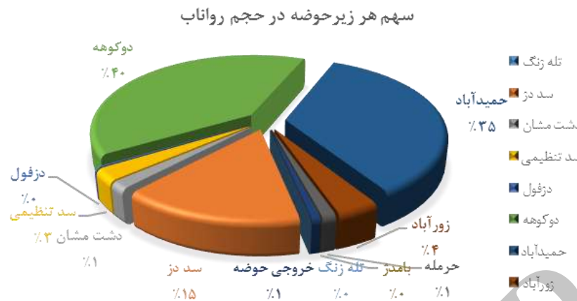
شکل ۱۴. میزان مشارکت هر زیرحوضه در سیل خروجی کل حوضه
