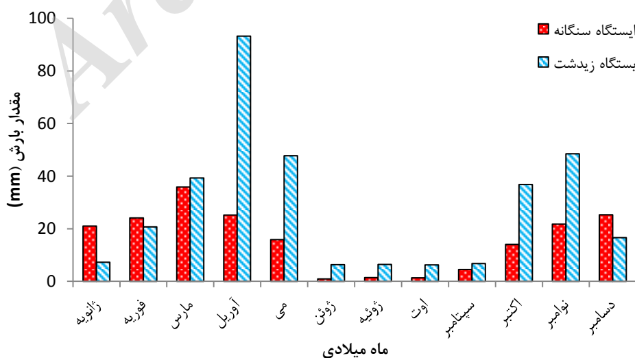
شکل ۲. میانگین ماهانه بارش در ایستگاه سنگانه و ایستگاه زیدشت (به طور تقریبی اولین ماه میلادی از دهم دی ماه و آخرین ماه میلادی از دهم آذرماه شروع می‌شود)
