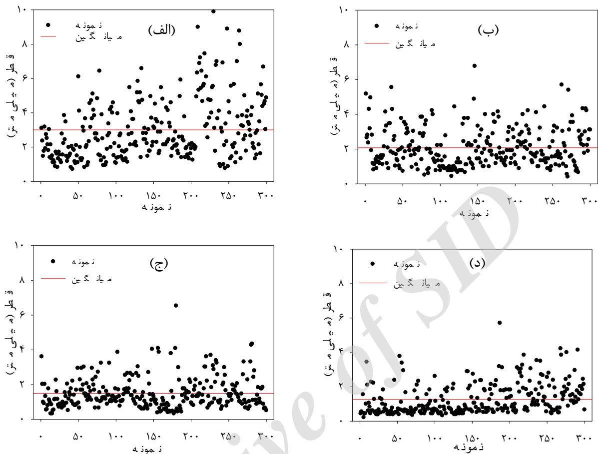
شکل ۷. اسکتر پلات توزیع قطرات بارش شبیه‌سازی شده در فشارهای ۲۰ (الف)، ۴۰ (ب)، ۶۰ (ج) و ۸۰ (د) کیلوپاسکال
