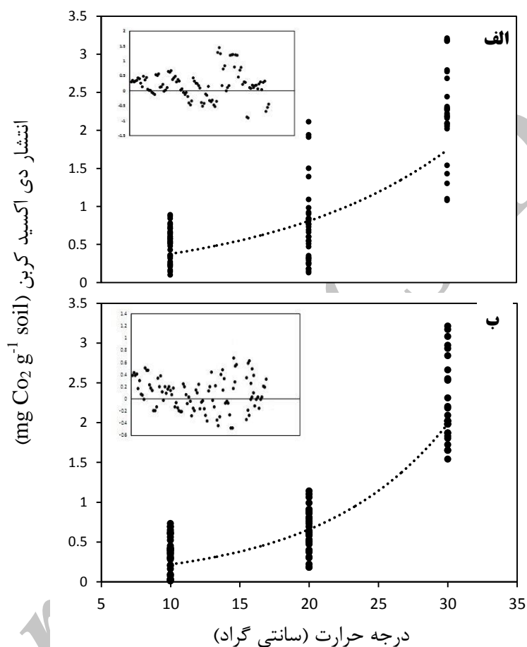
شکل ۱. برازش مدل آرهنیوس برای نمونه‌های خاک در دو اکوسیستم چرا شده (الف) و قرق (ب). نقاط براساس میزان تنفس خاک در سه سطح دمایی طی دوره انکوباسیون حاصل شده است. نمودار کوچک درج شده آنالیز اختلاف بین داده‌های اندازه‌گیری شده و شبیه‌سازی شده است.
