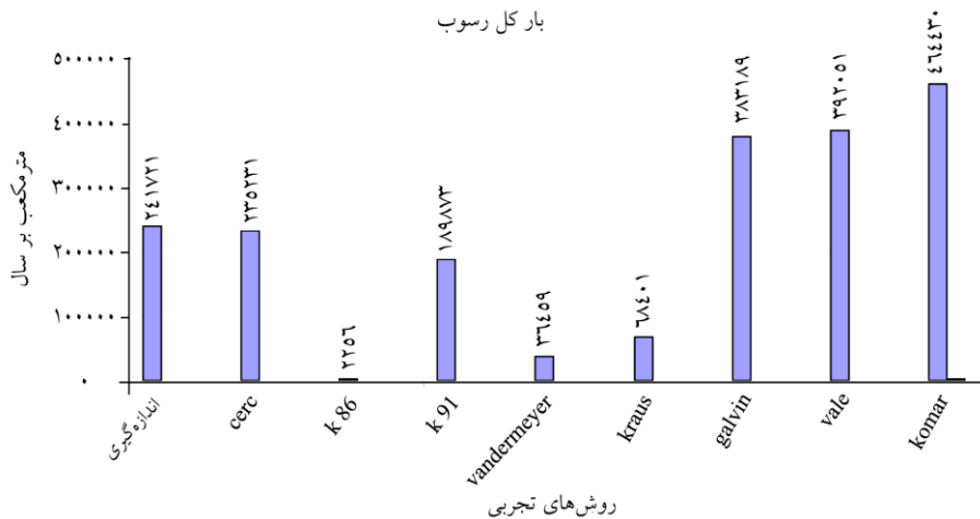
شکل 2- مقایسه نتایج روش های تجربی در برآورد انتقال رسوبات خور ریگ
