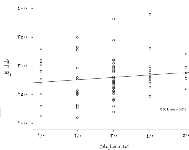
نمودار ۱- نمودار خطی پراکنش طول کل و تعداد ضایعات انگل لرنئا در ماهی کپور معمولی
