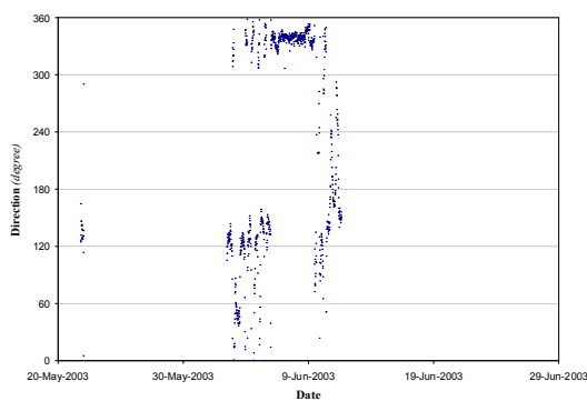
شکل ۲۶- سری زمانی تغییرات جهت جریان در ایستگاه C 5
