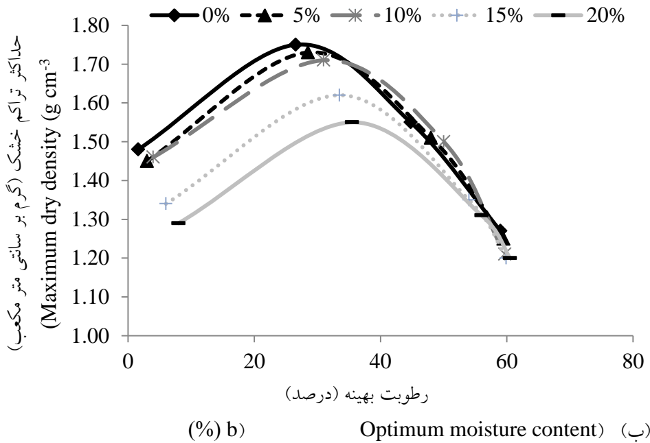
شکل ۸- منحنی حداکثر تراکم خشک خاک و رطوبت بهینه برای خاک‌های تیمار شده با خاکستر در زمان عمل‌آوری ۱۴ روز. Figure 8. Maximum dry density-water content curve for soil treated by ash in curing time of 14 day.
