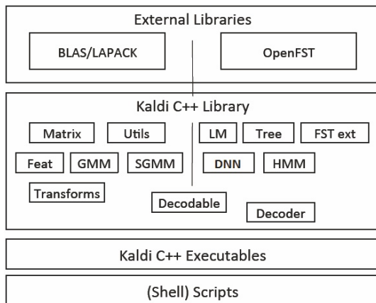
(شکل-1): نمایی ساده‌شده از اجزای نرم‌افزاری سامانه کلدی (Figure-1): A simplified diagram on the software modules from the Kaldi toolkit
