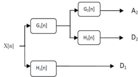
(شکل-۲): روش بانک فیلتر در تجزیه سیگنال x[n] به زیر باندهایش
