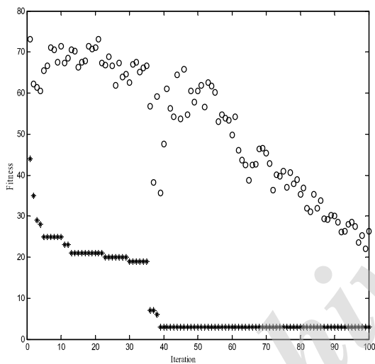
(شکل-۷): نمونه‌ای از اجرای الگوریتم پیشنهادی جهت طبقه‌بندی دو کلاس S و ZNF
