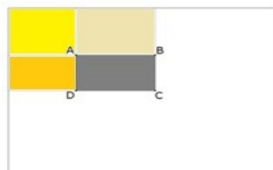
(شکل-۶): محاسبه مجموع مقادیر پیکسلی یک ناحیه در روش تصاویر انتگرالی
