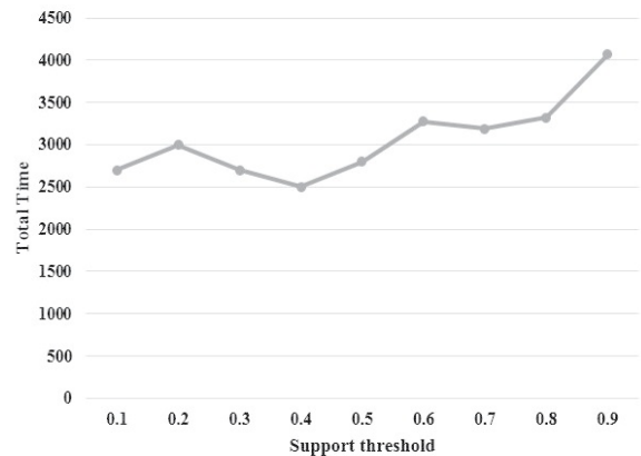
(شکل-۶): زمان کل در برابر تغییرات حد آستانه پوشش
