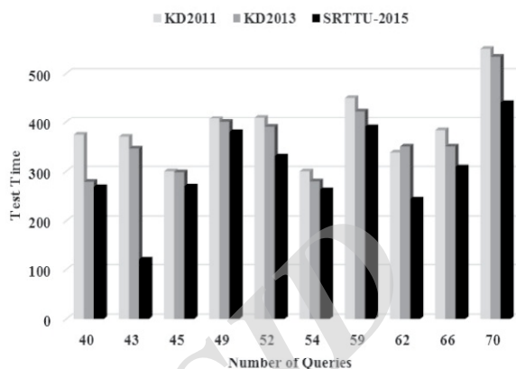
(شکل-۹): مقایسه زمان تست با افزایش تعداد پرس‌وجوها
