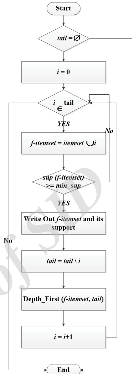
(شکل-۵): نمودار جعبه ای تابع اول عمق
