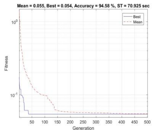
(شکل-۹): بهترین و میانگین اجرای الگوریتم ازدحام ذرات جهت بهینه‌سازی پارامترهای سیستم فازی سوگنو (Figure-9): The Best and Average Fitness of the PSO for Optimization of Sugeno Fuzzy Inference Model
