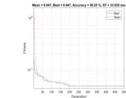
(شکل-۱۱): بهترین و میانگین اجرای الگوریتم مبتنی بر جغرافیای زیستی جهت بهینه‌سازی پارامترهای سامانه فازی سوگنو (Figure-11): The Best and Average Fitness of the Biogeography Algorithm for Optimization of Sugeno Fuzzy Inference Model
