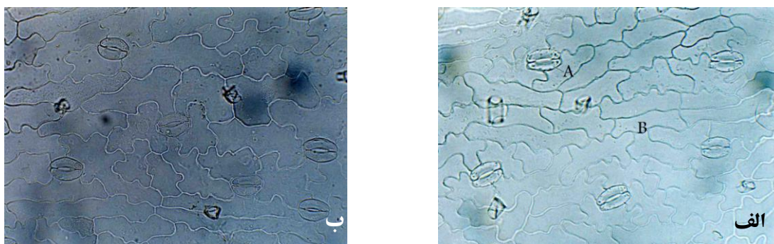
شکل ۲- نمایی از بشره برگ درمنه دشتی. الف) رویشگاه طبیعی؛ ب) مزرعه (بزرگنمایی ۲۰). A: سلول روزنه؛ B: بشره
