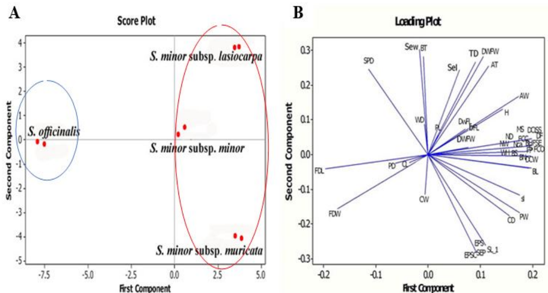
شکل ۴- نمودار رسته‌بندی گونه‌ها روی مؤلفه‌های اصلی اول و دوم- نمودار بارگذاری گونه‌ها (A) و نمودار بارگذاری صفات (B): H (نوع کرک: کرک خوابیده، راست و موج‌دار (۰) و افراشته، راست (۱))، WH (کرک روی باله: بدون کرک (۰) و دارای کرک (۱))، BH (کرک روی بدنه: بدون کرک (۰) و دارای کرک (۱))، PL (طول کرک)، PD (فاصله بین کرک (μm))، S (شکل بذر: مخروطی (۰)، کوزه‌ای (۱) و تخم‌مرغی (۲))، BT (ضخامت ناحیه ۱/۳ زیرین (mm))، AT (ضخامت ناحیه ۱/۳ بالایی (mm))، SPD (عمق حفره (mm))، CW (عرض حفره (mm))، CL (طول حفره (mm))، WFW (عرض چین‌خوردگی (mm))، DWFL (طول چین‌خوردگی (mm))، BFL (طول ناحیه بدون چین‌خوردگی پایین (mm))، FP (الگوی چین‌خوردگی)، EPSC (الگوی سلول‌های اپیدرمی: مشبک (۰) و راه‌راه (۱))، AW (دیواره آنتی‌کلینال: فرورفته (۰)، چروکیده (۱)، فرورفته - چروکیده (۲) و برجسته (۳))، PW (دیواره پری‌کلینال: فرورفته (۰) و چروکیده (۱))، EPS (شکل سلول اپیدرمی: چندضلعی نامنظم - مستطیلی (۰) و طولی (۱))، SEP (تزیینات سطح: مشبک (۰)، راه‌راه (۱) و حفره‌دار (۲))، MS (نوع موم: لایه‌ای صاف - گرانول - صفحات کوچک (۰)، پوسته‌پوسته و گرانول (۱))، NW (تعداد باله: ۲ باله (۰) و ۴ باله (۱))، WD (ضخامت باله (mm))، DCW (تعداد برگه درونی: یک برگه (۰) و دو برگه (۱))، BN (تعداد برگه بیرونی: یک برگه (۰) و دو برگه (۱))، BL (طول برگه بیرونی (mm))، NC (تعداد کاسبرگ)، DCL (طول کاسبرگ (mm))، DCW (عرض کاسبرگ (mm))، BS (شکل برگه بیرونی: واژ تخم‌مرغی (۰)، سرنیزه‌ای - تخم‌مرغی (۱)، و سرنیزه‌ای (۲))، SL (طول خامه (mm))، SS (شکل کلاله: نخ‌مانند - زگیل‌دار (۰) و قلم‌موم‌مانند (۱))، DEpi (ابعاد کاسبرگ بیرونی (mm))، FCC (رنگ گل باز شده: سبز و قسمت بالایی ارغوانی (۰) و سبز و کم‌رنگ با لکه‌های ارغوانی (۱))، FCO (رنگ غنچه‌ها: ارغوانی - قهوه‌ای (۰) و سبز با حاشیه ارغوانی (۱))، FDL (طول گل آذین (mm))، FDW (عرض گل آذین (mm))، DF (قطر گل (mm))، FSE (جنسیت گل: نر (۰)، ماده (۱) و نر - ماده (۲))، SeL (طول بذر (mm))، SeW (عرض بذر (mm))، NCa (تعداد برچه: یک برچه (۰) و دو برچه (۱))، SS (شکل کلاله: نخ‌مانند - زگیل‌دار (۰) و قلم‌موم‌مانند (۱)) و ND (تعداد خامه: یک خامه (۰) و دو خامه (۱))
