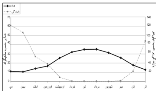
شکل ۱- منحنی باران دمایی منطقه حفاظت شده ارژن-پریشان
