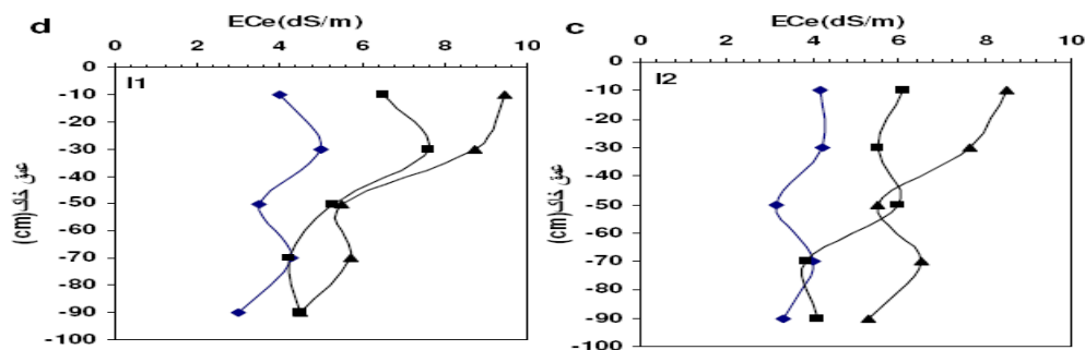
شکل ۴- میانگین فصلی شوری در پروفیل خاک در تیمارهای I 1 , I 2 , I 3 , I 4
