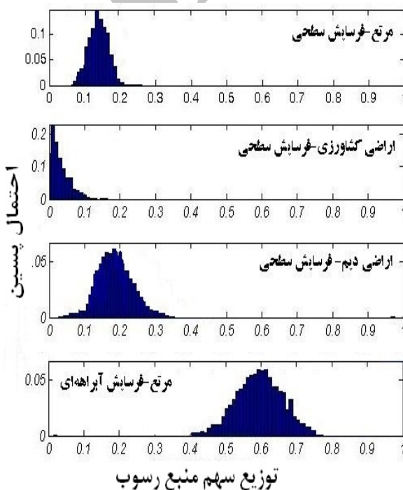
شکل ۴- برآورد سهم چهار منبع رسوب حوضه آبخیز زیدشت با استفاده از مدل عدم قطعیت
