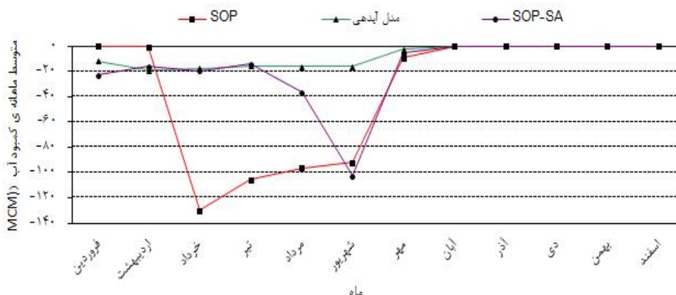
شکل ۶- متوسط ماهانه کمبود آب در سه مدل در بازه زمانی ۱۳۵۵-۱۳۵۶.
