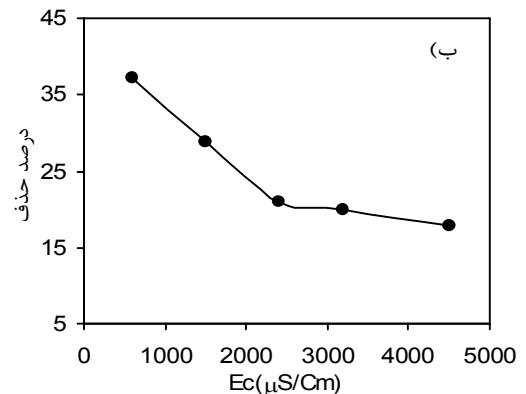
شکل ۲- اثر شوری بر میزان جذب کادمیم در واحد جرم کربنات کلسیم (الف) و درصد حذف آن (ب)
