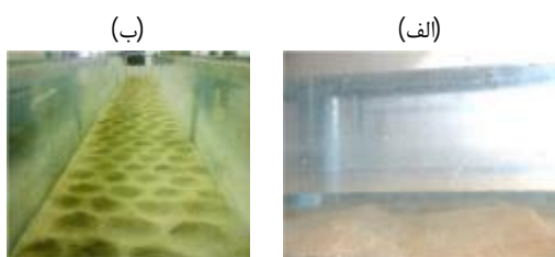
شکل ۲- نمایشی از شکنج‌های پولکی و موازی در کف فلوم آزمایشگاهی و موقعیت سرعت سنج ADV، الف- شکنج موازی، ب- شکنج پولکی
