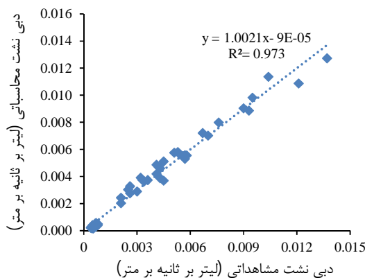
شکل ۵- مقایسه مقادیر محاسباتی و اندازه‌گیری شده دبی نشت در مرحله آموزش
