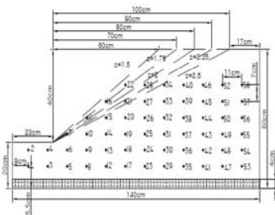
شکل ۱- طرح شماتیک مدل آزمایشگاهی و محل قرارگیری پیژومترها
