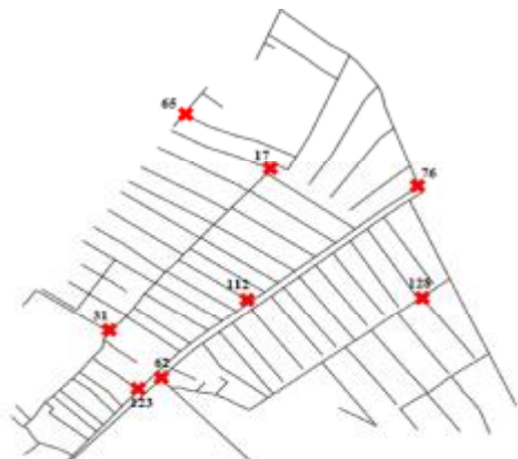
شکل ۴- محل گره‌های انتخاب شده برای اندازه‌گیری میدانی فشار آب در شهرک بزین
