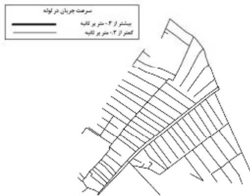
شکل ۸- توزیع سرعت جریان عبوری از لوله‌های شبکه توزیع آب شهرک بزین در ساعت ۴ روز اول دی سال ۱۳۹۱
