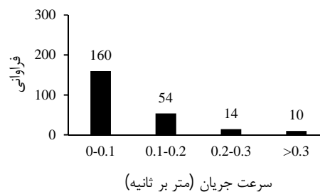
شکل ۶- هیستوگرام فراوانی میانگین سرعت جریان عبوری از لوله‌های شبکه توزیع آب شهرک بزین در ماه مرداد سال ۱۳۹۱
